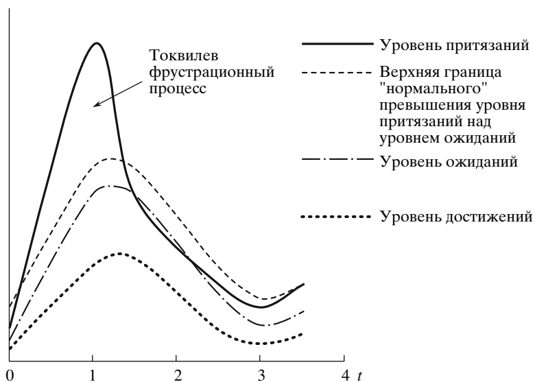
Рис. 2. Гипотетическая картина развития токилевского фрустрационного процесса ("драматический" вариант).
