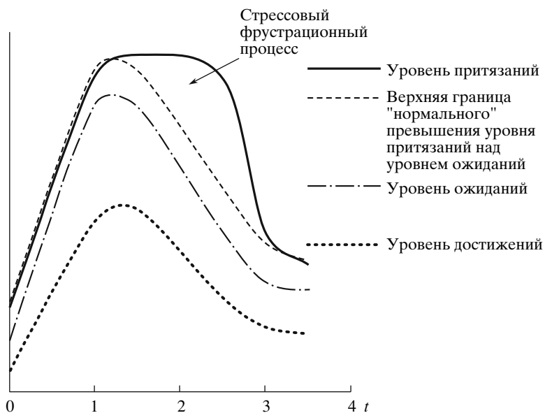
Рис. 1. Гипотетическая картина развития стрессового фрустрационного процесса. Примечание: Здесь и в рисунках 2 и 3 я никак не обозначаю размерность оси Y , потому что таких размерностей может быть много. В простейшем случае изображенные на графике показатели могут оцениваться в денежной форме. Тогда роль размерности оси Y будет играть та или иная денежная единица.
